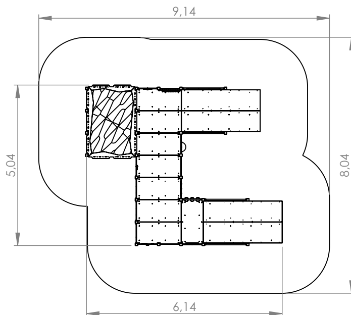
Parametry wysokościowe
